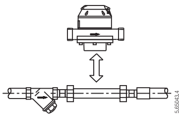
Zähler mit Gewindeanschluss
